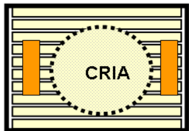
Langstroth o Dadant (vist des de dalt)
